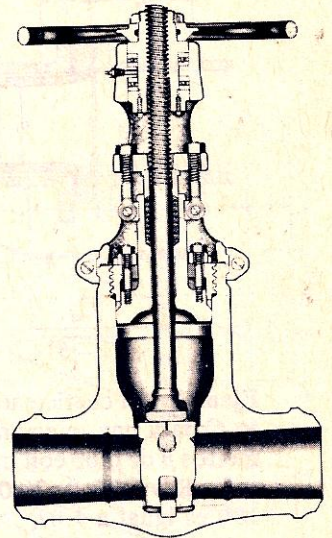
Válvula de compuerta de cuña flexible (tapa con sello a presión)
