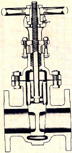
Válvula de compuerta de cuña (tapa atornillada)
