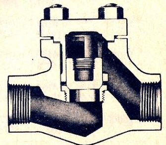
Válvula de retención de paso recto, con obturador ascendente
